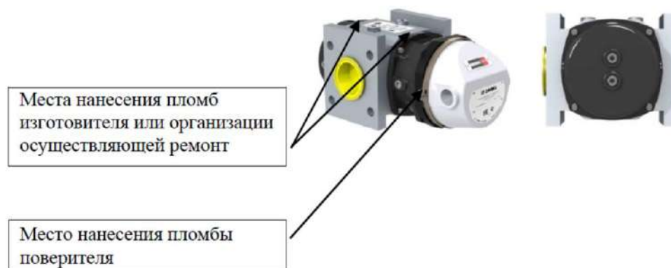
Рисунок 1.9 – Схема пломбирования счетчика
