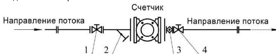
Рисунок 2.8 – Установка счетчика без перепускной линии
