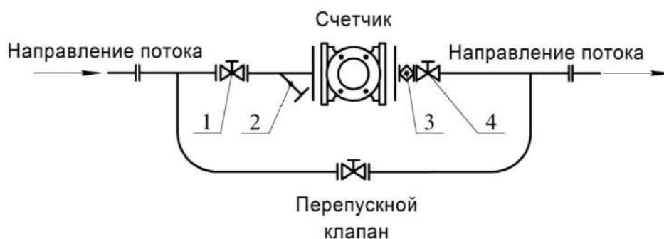
Рисунок 2.5 – Горизонтальная установка счетчика 1, 4 – изолирующие клапаны, 2 – фильтр, 3 – компенсатор
