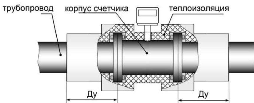
Рисунок 2.6 – Теплоизоляция счетчика
